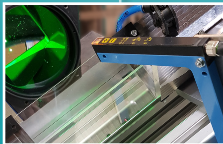
Glasrutsche mit verstellbarer Neigung
